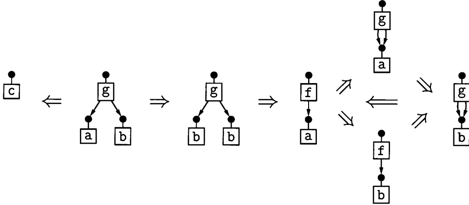
FIG. 12. Nonconfluence of \Rightarrow .
