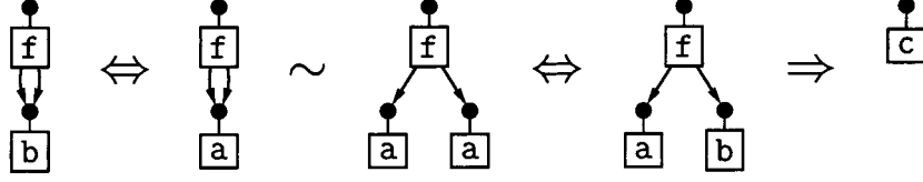
FIG. 7. Confluence without confluence modulo \sim .
